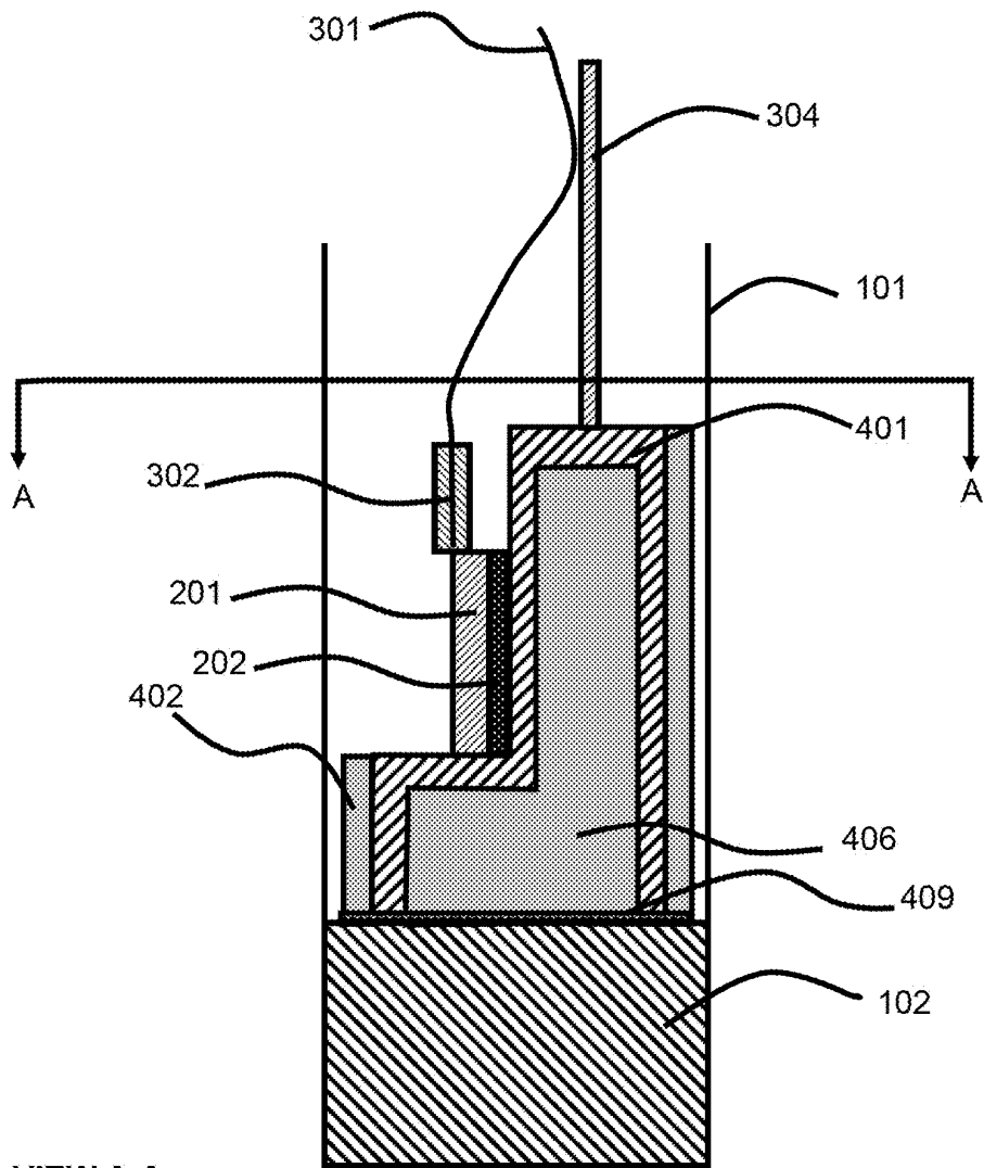
VIEW A-A
