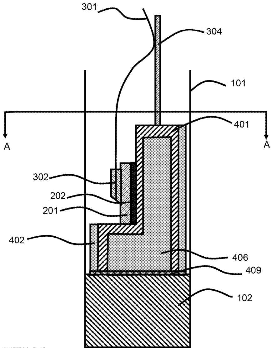
VIEW A-A
