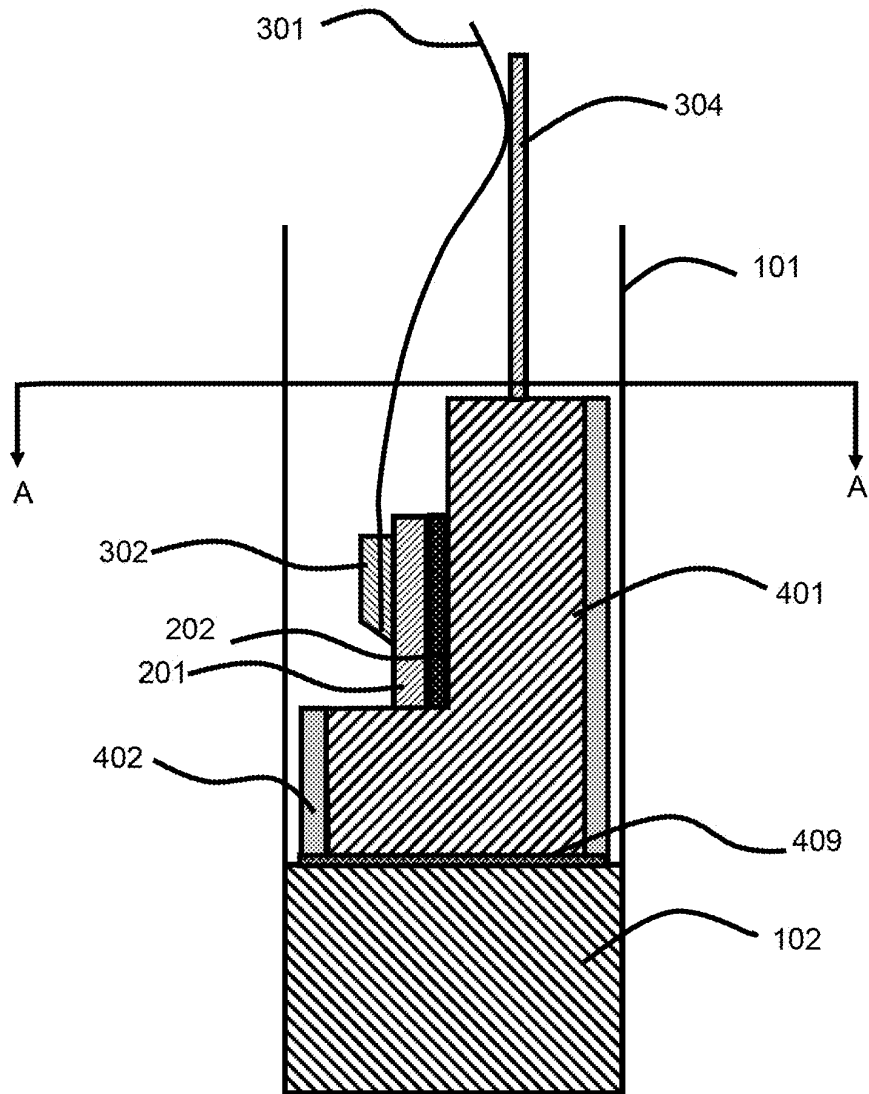
VIEW A-A
